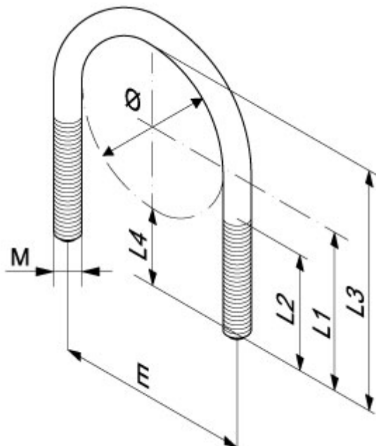
Fig.112 Krambeugel zwaar, Thermisch verzinkt
