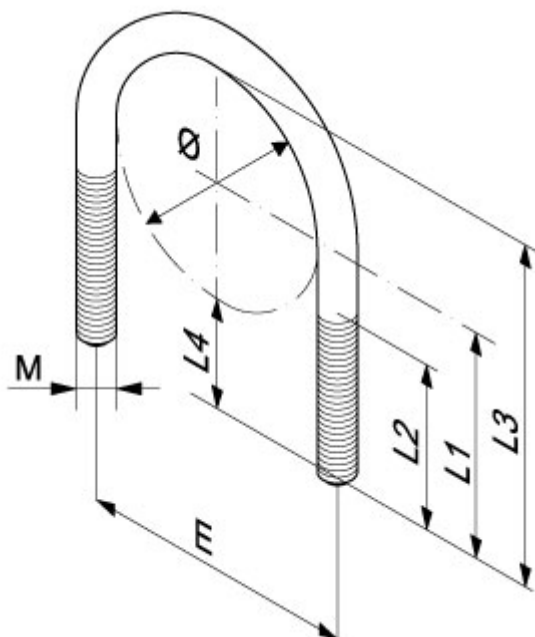
Fig.115 Krambeugel DIN3570, Electrolytisch verzinkt
