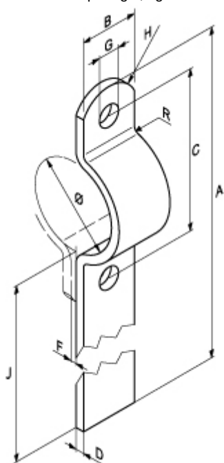
Fig.116 Staartbeugel, S235 zwart
