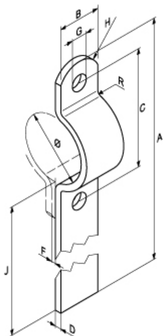
Fig.116 Staartbeugel, RVS-304
