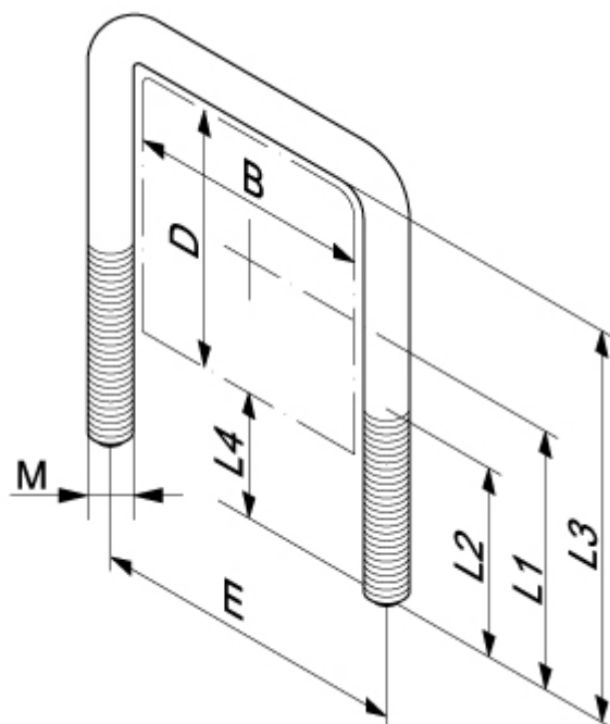
Fig.117 Rechthoekkram, Electrolytisch verzinkt
