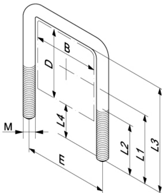
Fig.117 Rechthoekkram, Thermisch verzinkt
