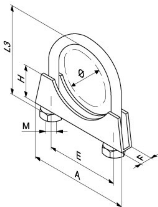
Fig.119 Uitlaatbeugel, RVS-316
