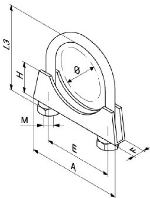
Fig.119 Uitlaatbeugel, RVS-304
