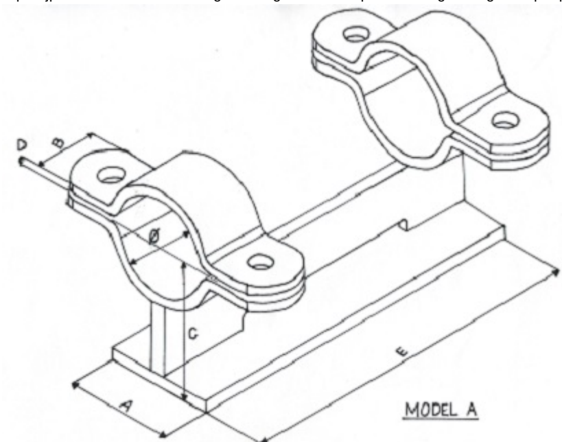
Fig.127 Pijpschoen RVS, RVS-304
