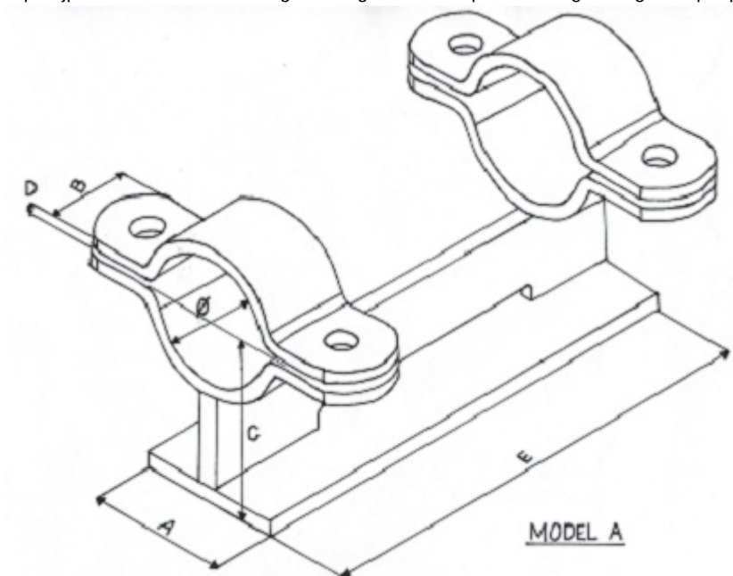
Fig.127 Pijpschoen RVS, RVS-316
