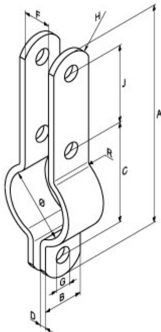
Fig.132 3-gatsbeugel middenzwaar, Thermisch verzinkt
