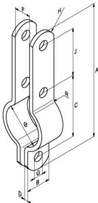
Fig.132 3-gatsbeugel middenzwaar, S235 zwart
