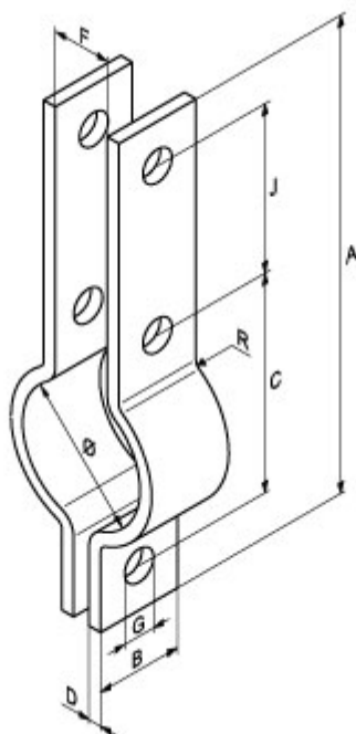
Fig.134 3-gatsbeugel zwaar, S235 zwart
