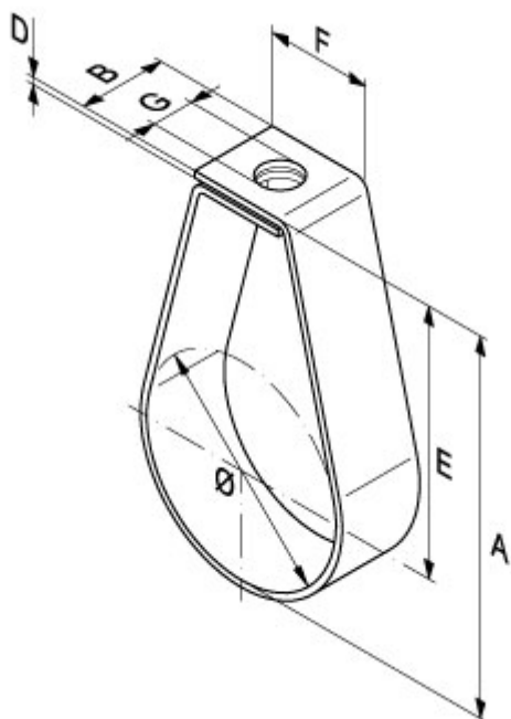
Fig.136 Hangbeugel schuivend, Thermisch verzinkt
