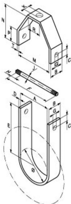
Fig.138 Hanger v. isolatie, Thermisch verzinkt
