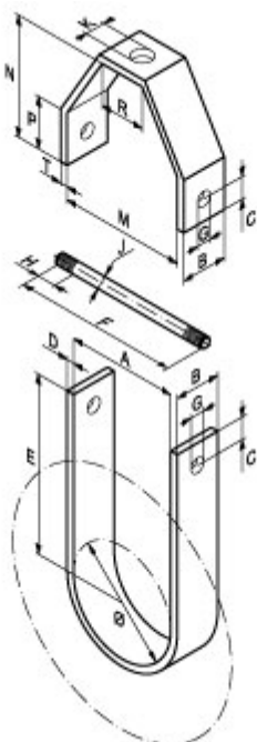
Fig.138 Hanger v. isolatie, S235 zwart
