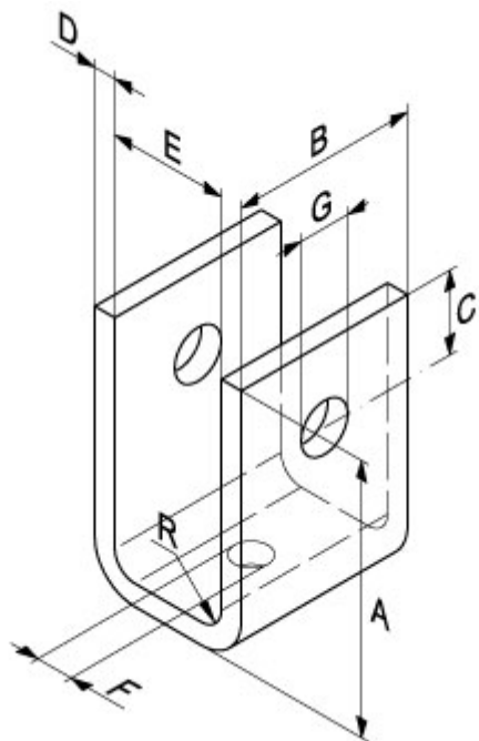
Fig.140 Ophangbeugel, Thermisch verzinkt
