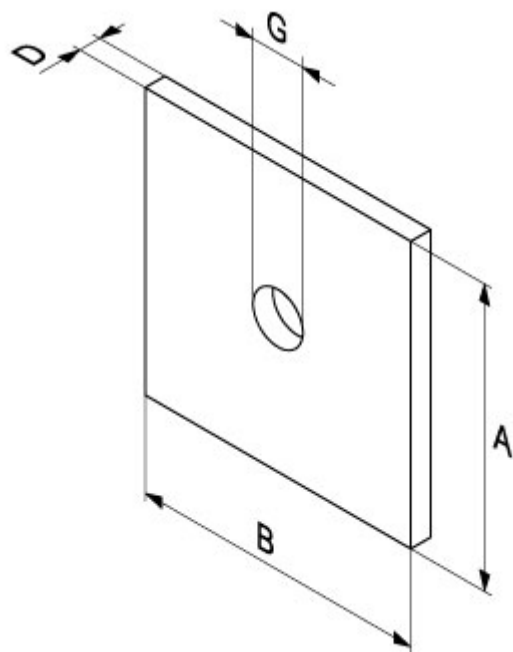
Fig.142 Vierkante sluitplaat, RVS-304
