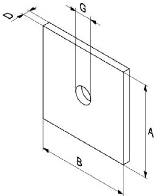
Fig.142 Vierkante sluitplaat, S235 zwart
