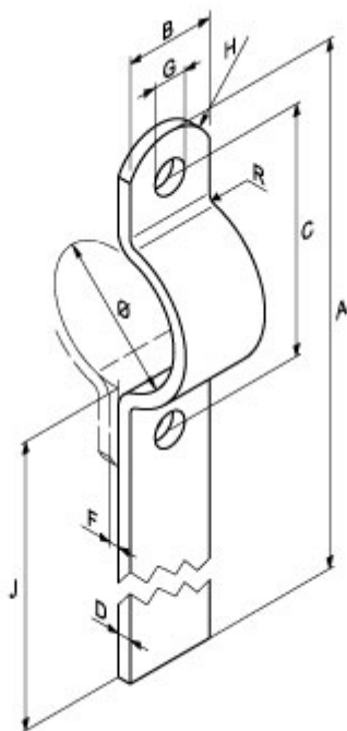
Fig.149 Staartbeugel (146), RVS-316
