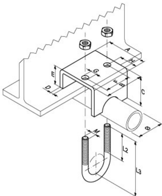
Fig.170 Profielbeugel, Thermisch verzinkt
