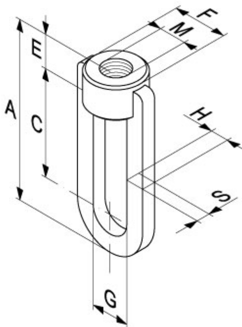
Fig.200 Oogmoer, Thermisch verzinkt
