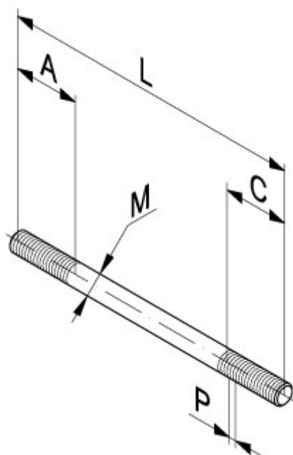
Fig.207 Tapeind L+R, Thermisch verzinkt
