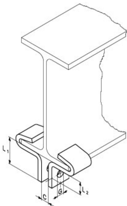
Fig.210 Balkklem, Thermisch verzinkt
