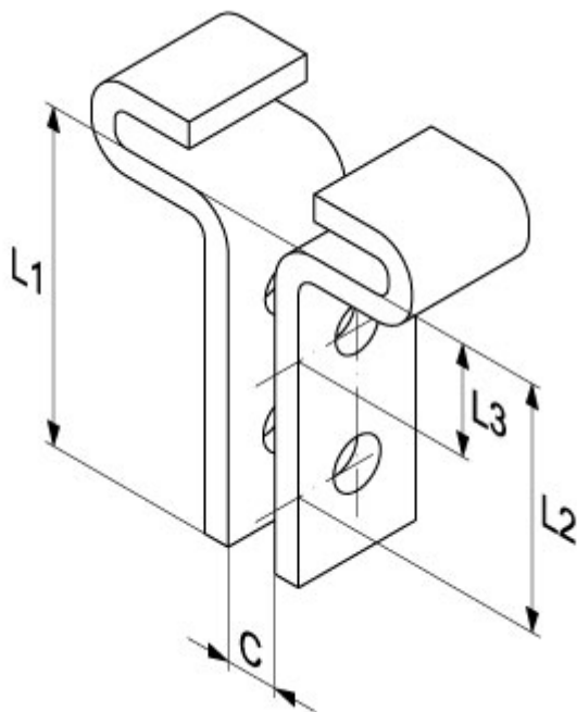
Fig.213 Balkklem, Thermisch verzinkt
