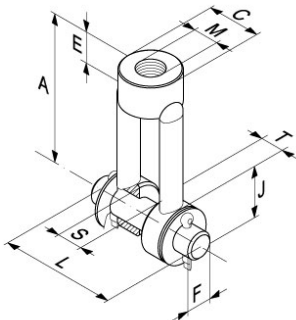
Fig.214 Gaffel, Electrolytisch verzinkt
