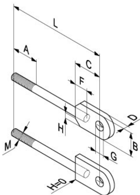
Fig.215 Ophangstang (plaat), S235 zwart
