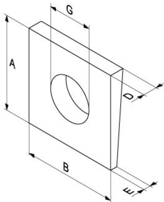
Fig.224 Hellingplaat DIN434, Thermisch verzinkt
