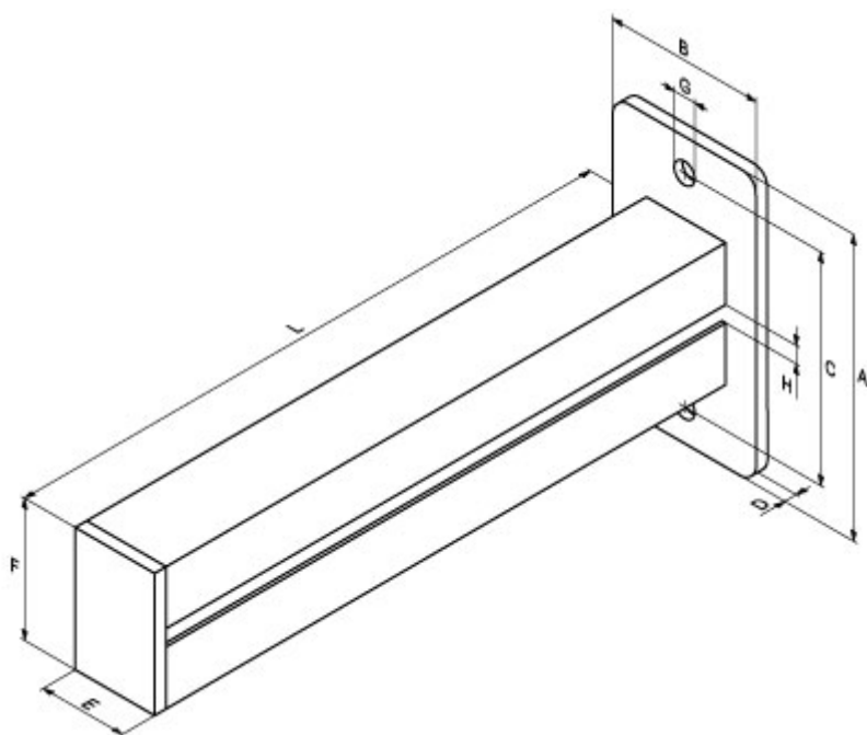
Fig.V , Thermisch verzinkt
